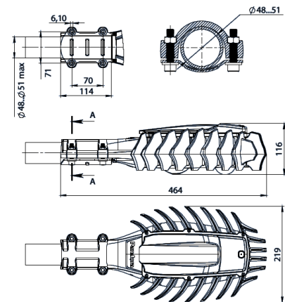
Рисунок 3. Габаритный чертеж
